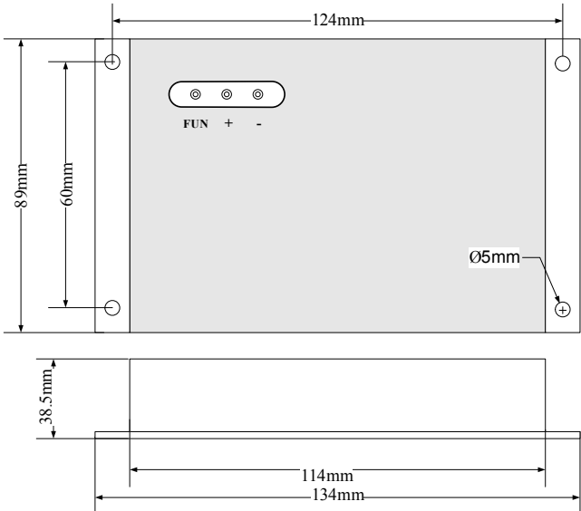
图 3-6-1 MCTC-CHM-B 尺寸图
