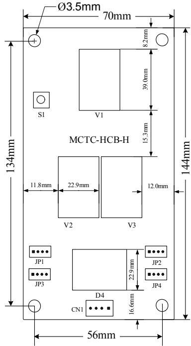
图3-3-10 安装尺寸
