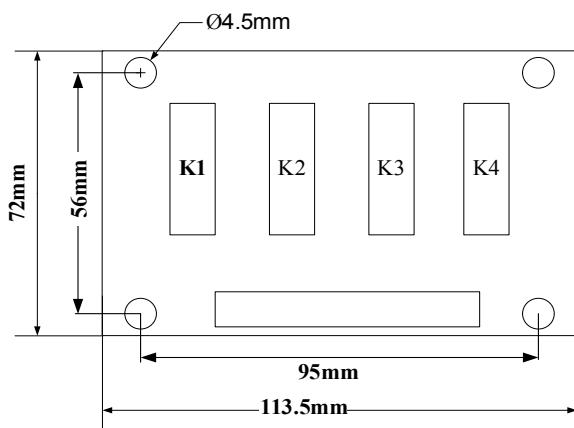
图3-5-2外观尺寸图
