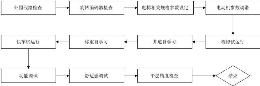
图7-1 调试流程
