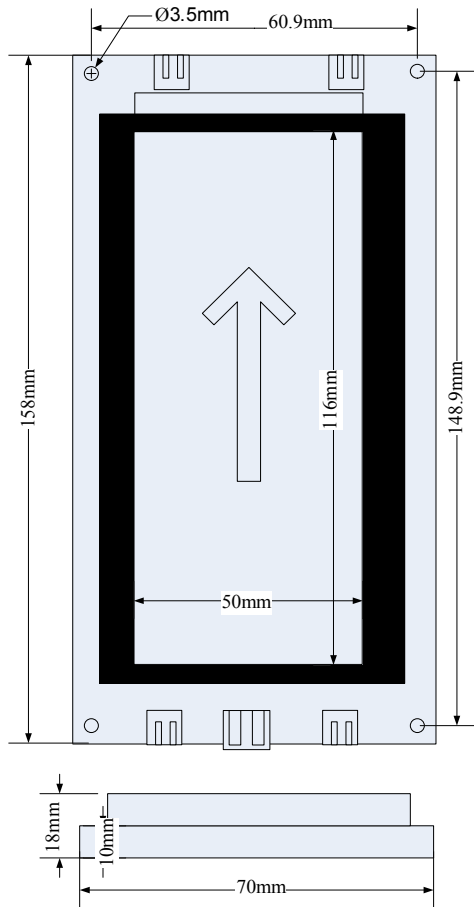
图3-3-6 MCTC-HCB-D1尺寸图
