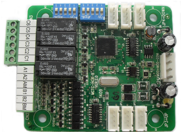
图 3-3-1 MCTC-HCB-B实物图
