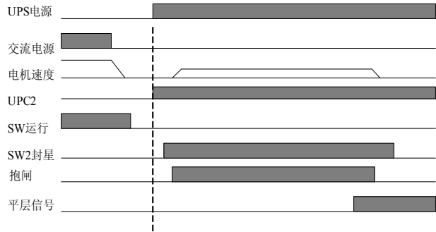
图7-5 自溜车时序
