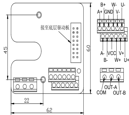
图4-6 MCTC-PG-B示意图
