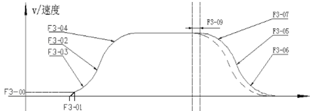
图6-4 速度曲线图
