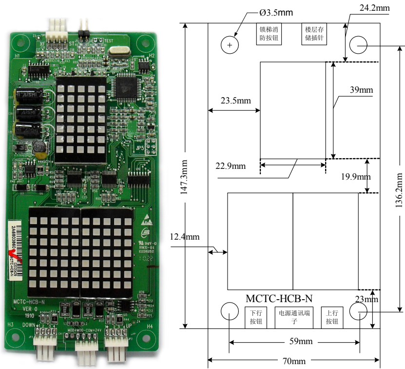
图3-3-13 MCTC-HCB-N实物图
