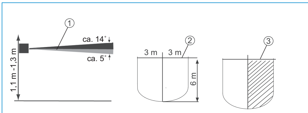
图 6：探测范围
