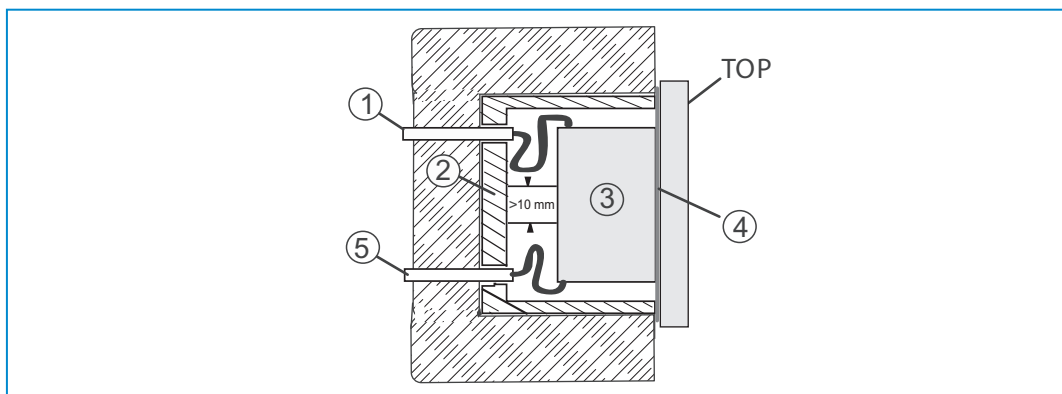
插图 7: SELV- 电路
