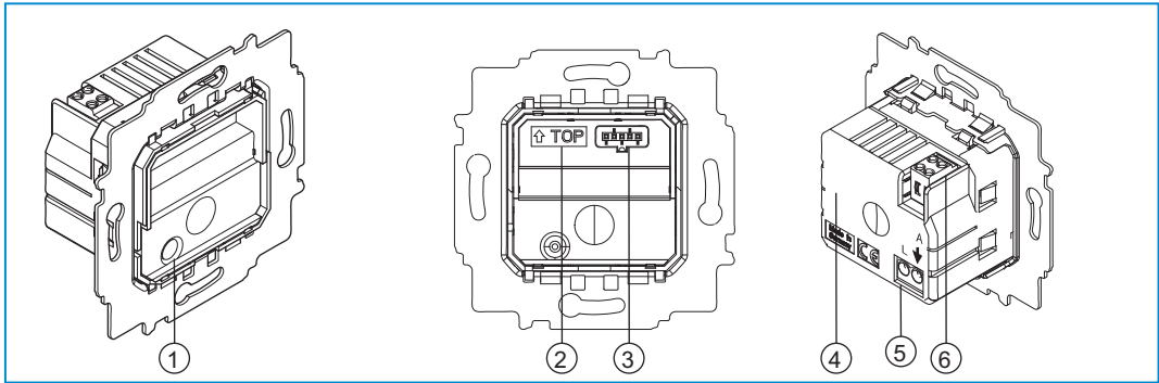
图 2：1 路运动检测器/开关执行器设备概览（无盖板）
